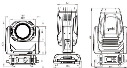
尺寸图
