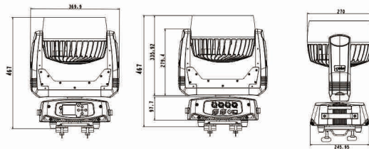
尺寸图
